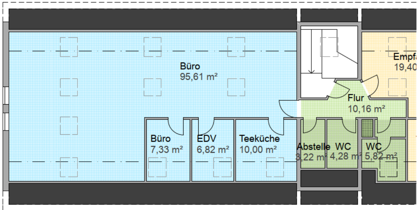
Grundriss DG - Teil 1 - M 1:100
