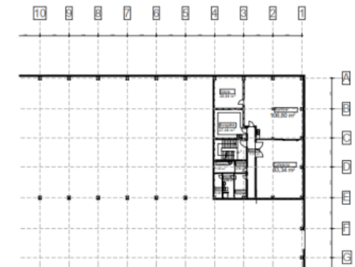
1. Obergeschoss M 1 : 200
