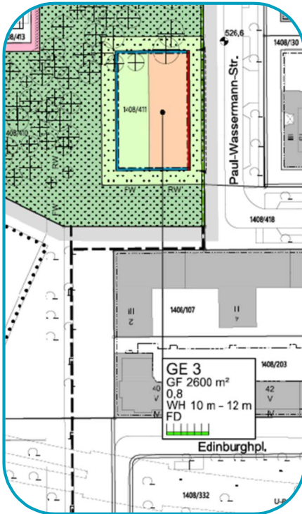
Auszug aus Bebauungsplan 1728d, Technologiepark Riem
