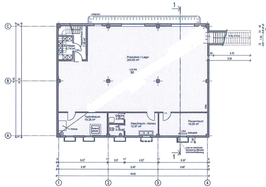
KELLERGESCHOSS
