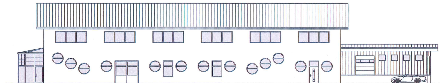
Ansicht Süd
