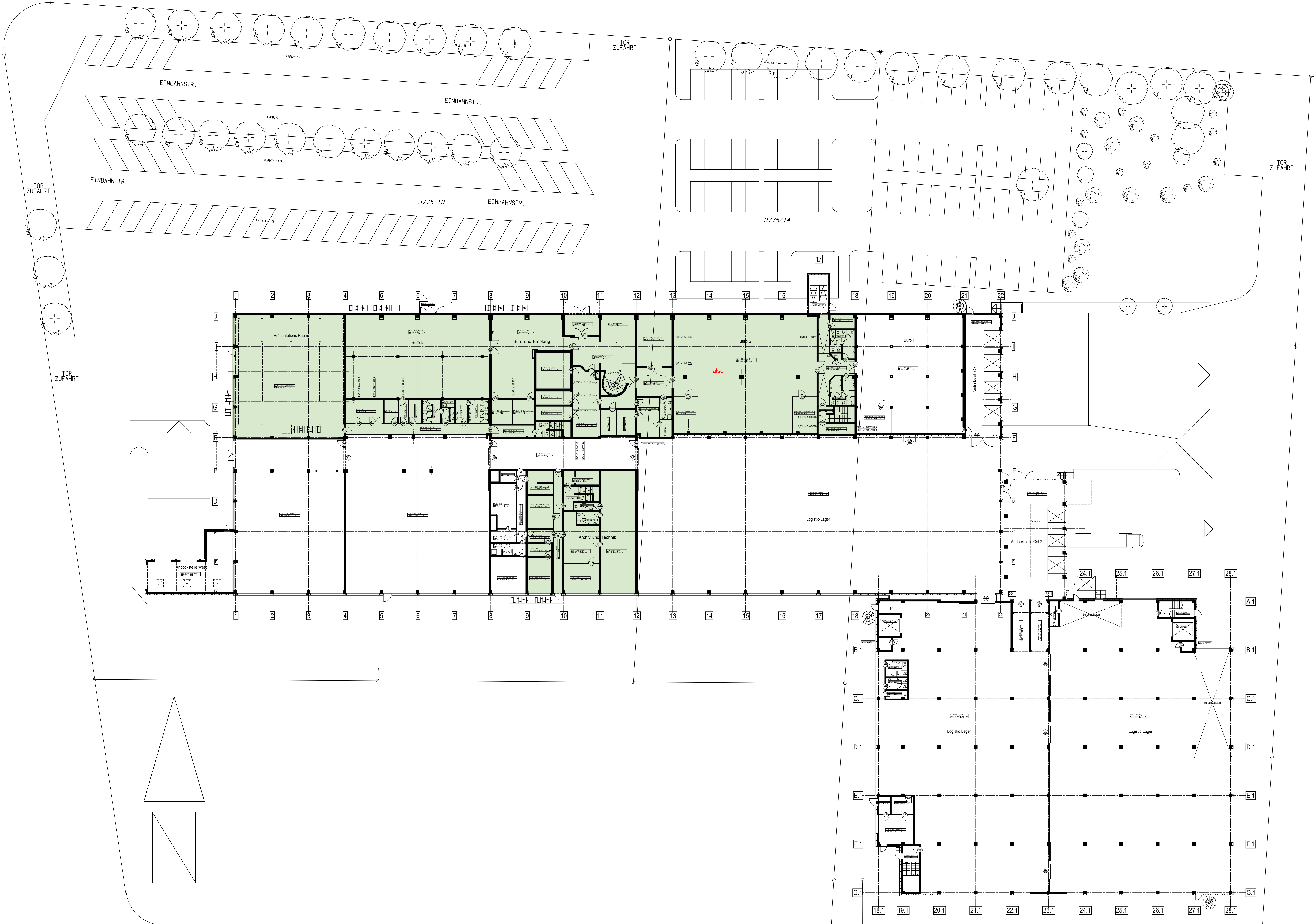
Objekt Ernst-Heinkel-Straße 4 Erdgeschoss mit Aussenanlagen M=1:200 Straubing, den 24.03.2015 STZ GmbH
