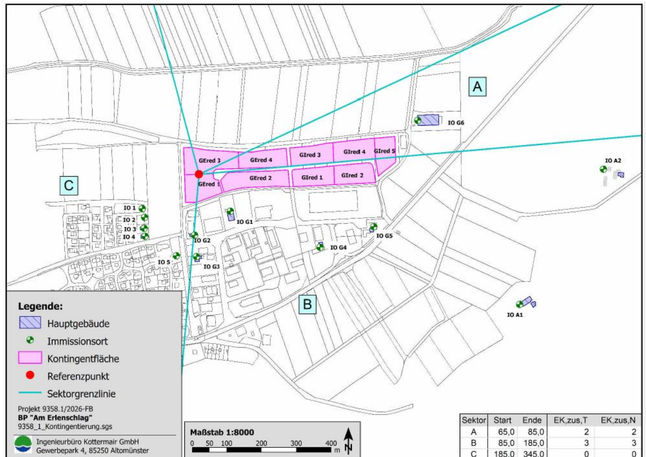
Abbildung 6: Immissionsorte und Zusatzkontingente (IB Kottermair 2026)
