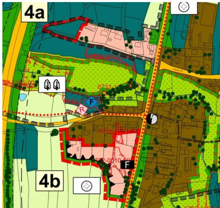
Darstellung Vorentwurf
