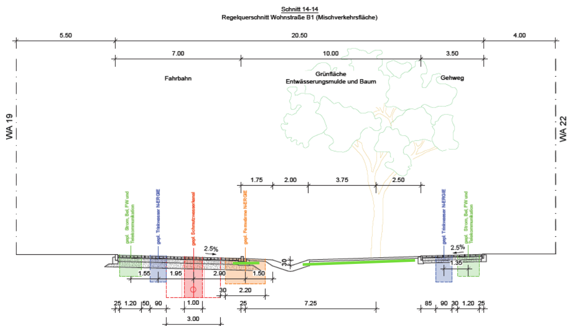
Abbildung 16 Querschnitt Wohnstraße B, (LP 2; Stand: 28.11.2025); Quelle: Gauff Engineering
