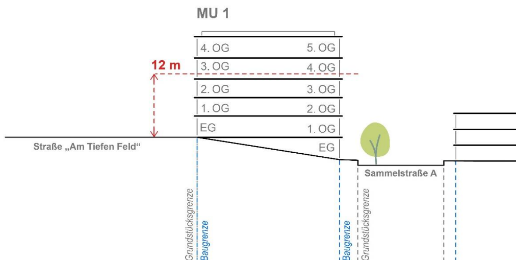
Abbildung 25: Schemaschnitt MU 1; Darstellung Höhenunterschied Sammelstraße A und Straße „Am Tiefen Feld“ © Stadt Nürnberg, Stadtplanungsamt
