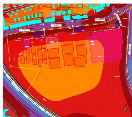
Abbildung 30 Links: Ohne Schallschutzwand entlang SWT (Lageplanskizze 7.3 des Gutachtens), rechts: Mit Schallschutzwand an SWT (Lageplanskizze 7.1) (Obermeyer, 05.06.2025); Kartengrundlage: Geobasisdaten © Bayerische Vermessungsverwaltung
