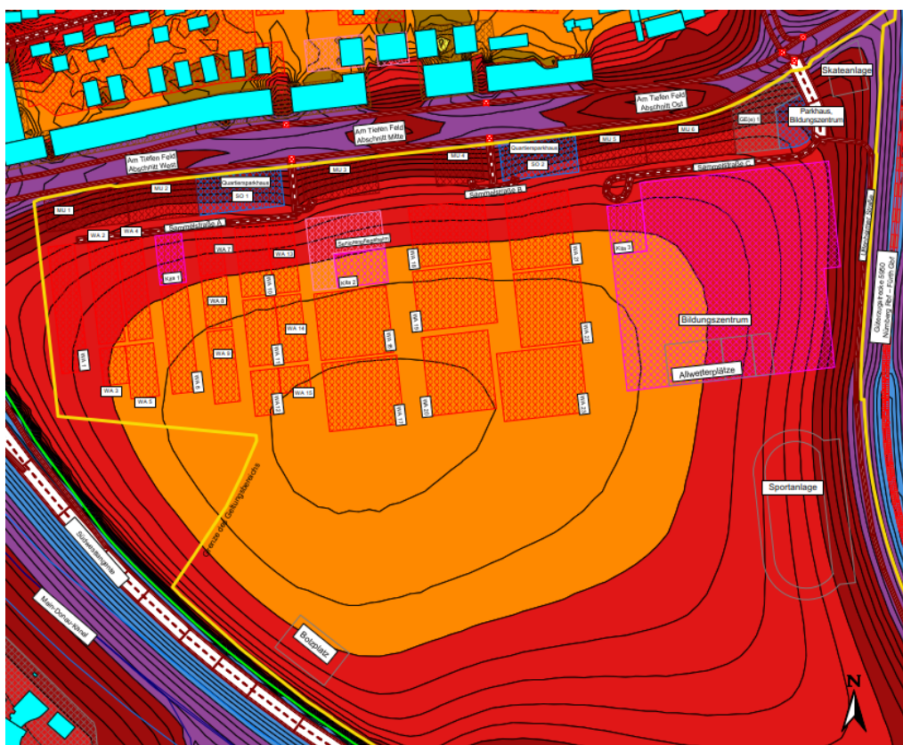
Abbildung 18 Freie Schallausbreitung Verkehrslärm mit Darstellung der Bauflächen (Obermeyer, 05.06.2025); Kartengrundlage: Geobasisdaten © Bayerische Vermessungsverwaltung
