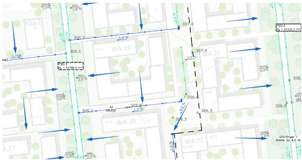
Abbildung 23: Entwässerungskonzept, Zoom-In, Entwässerung WA und Straßenverkehrsflächen, Henning Larsen (Fortschreibung Entwässerungskonzept 25.11.2025); Kartengrundlage: Geobasisdaten © Bayerische Vermessungsverwaltung
