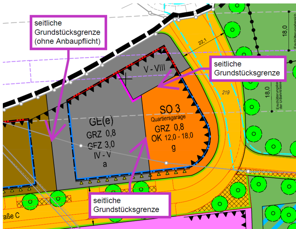
Abbildung 26: Erläuterung der Einordnung der seitlichen Grundstücksgrenzen am Beispiel des GE(e); Bebauungsplan, Arbeitsstand November 2025; Stadt Nürnberg; Kartengrundlage: Geobasisdaten © Bayerische Vermessungsverwaltung
