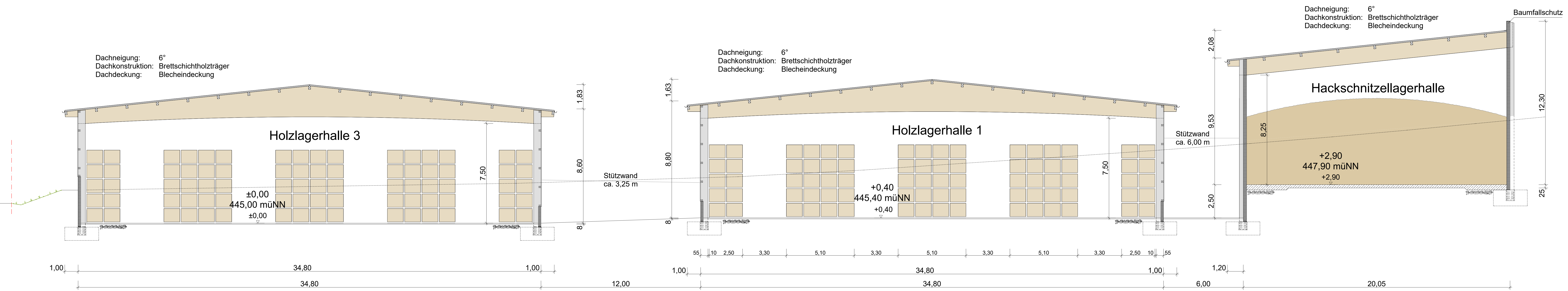
SCHNITT A-A
